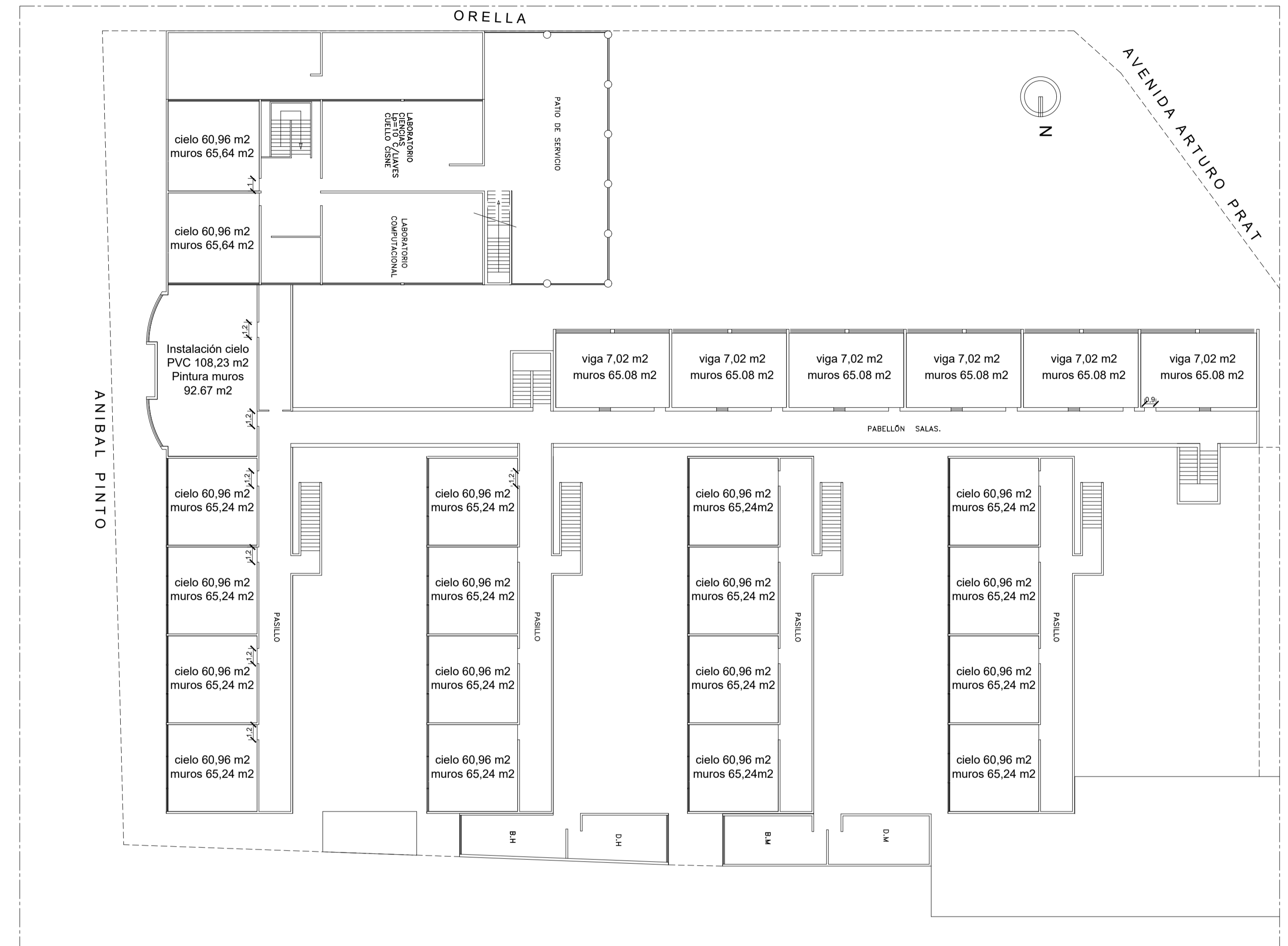
PLANTA SEGUNDO PISO ESCALA 1 : 400
