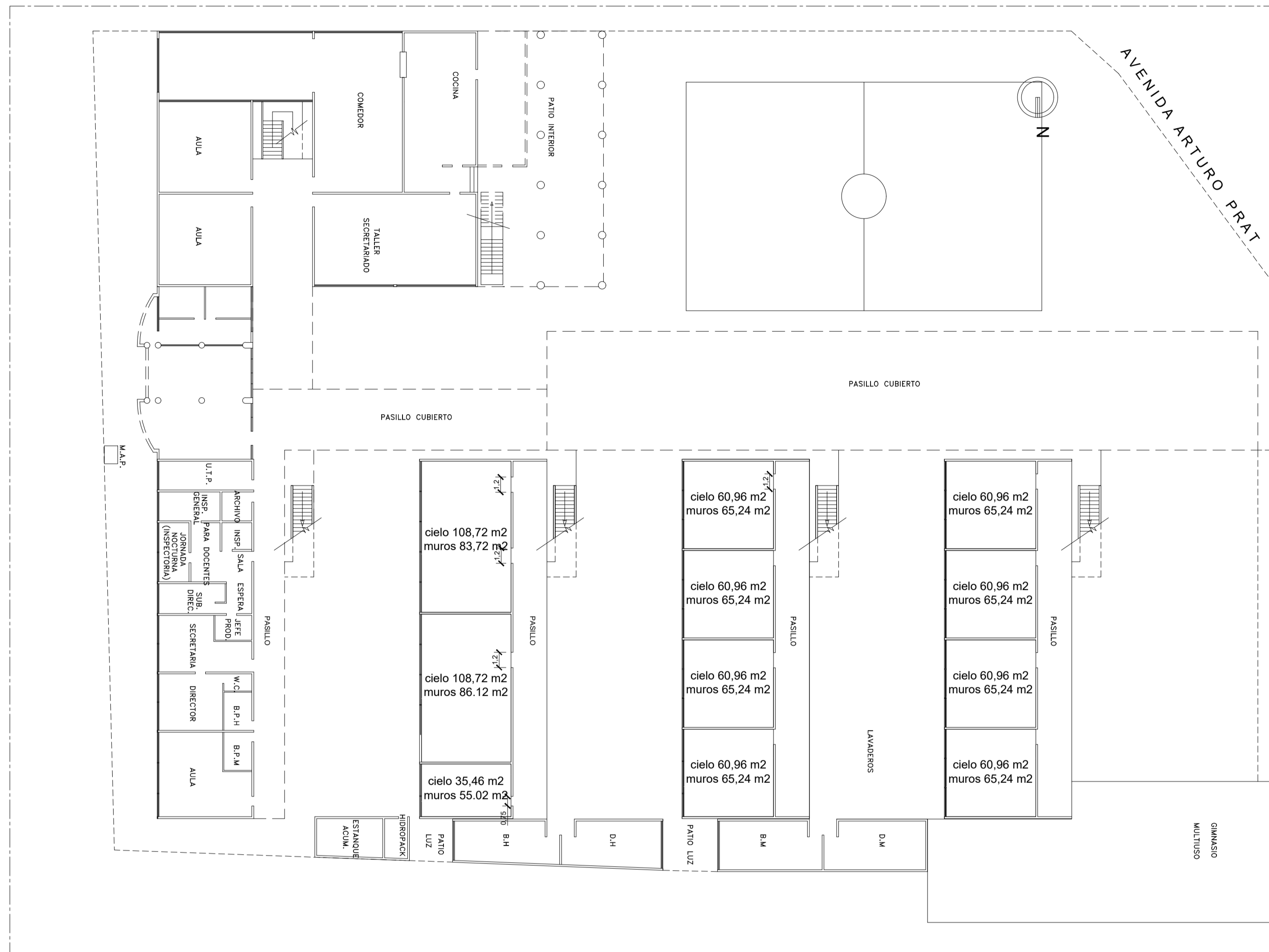
PLANTA PRIMER PISO ESCALA 1 : 400
