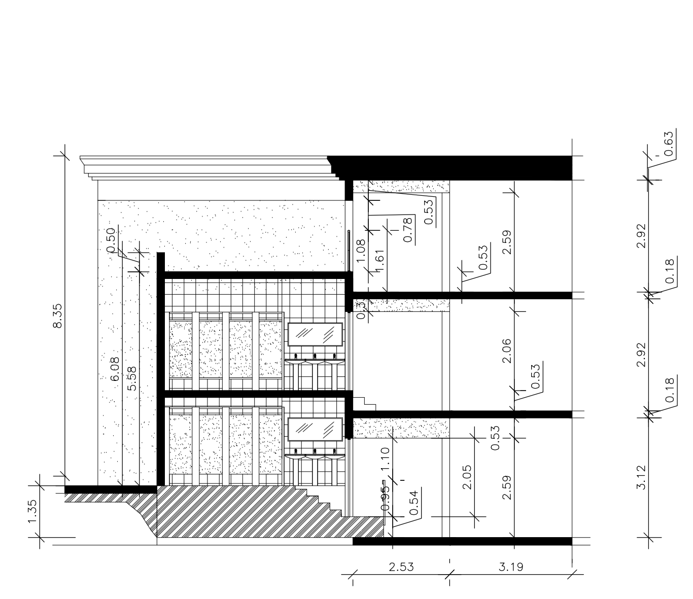
CORTE TIPO SITUACION PROYECTADA ESCALA 1:100
