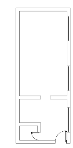
PLANTA SUBTERRANEO ESCALA 1 : 200
